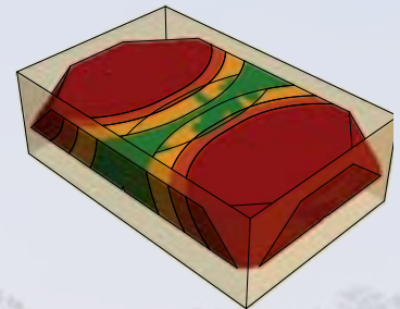
Effet de chaleur avec 2 côtés chauffés (format 6 x 4 m)
