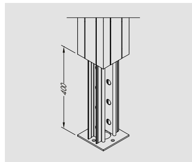
Pied de montage noyé
