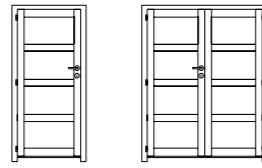
Porte vitrée 4V (simple et double) vitre claire ou acidifiée
