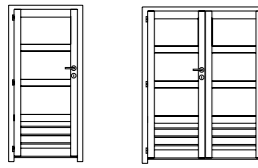
Porte vitrée 3V (simple et double) vitre claire ou acidifiée
